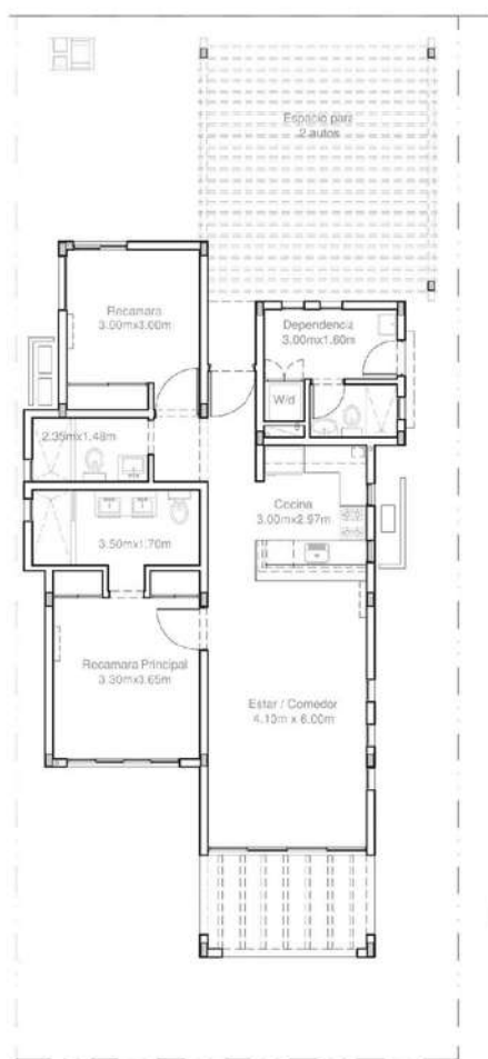
MODELO A 2 recámaras, 2 baños cuarto y baño de servicio 124 m 2
