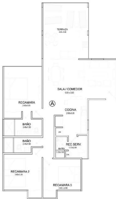
PLANTA 1, 2 3 recámaras, 2 baños, balcón cuarto y baño de servicio 122 m 2
