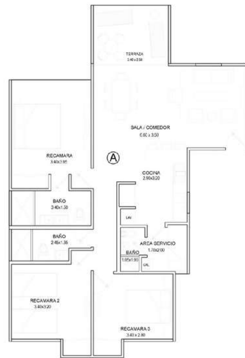
PLANTA 3, 4, 5 y 6 3 recámaras, 2 baños, balcón cuarto y baño de servicio 111 m 2
