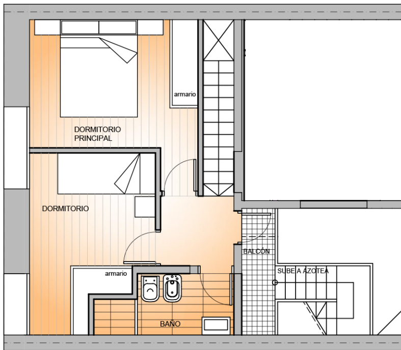
UNIDAD 001 - PLANTA ALTA
