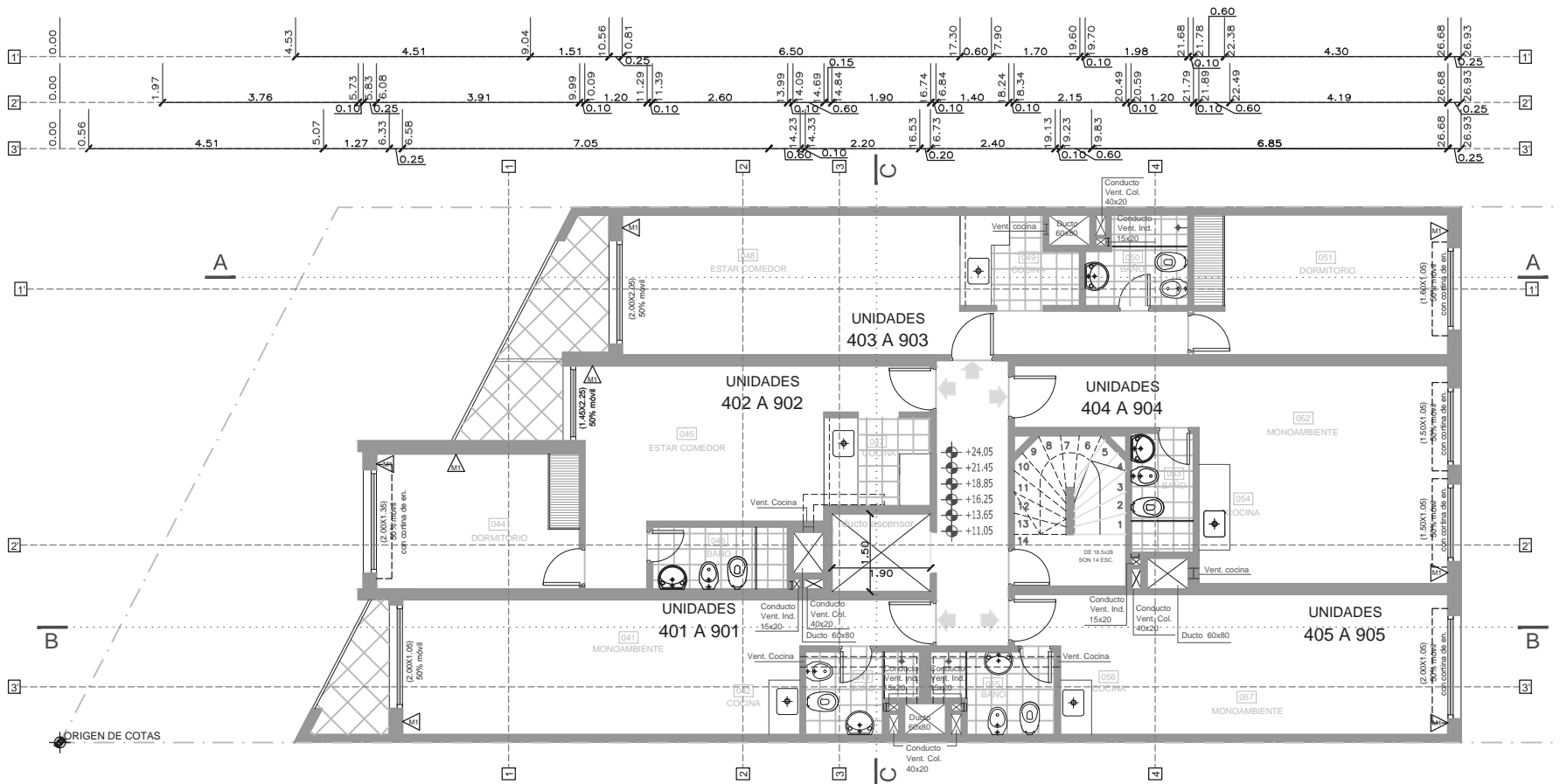
PLANTA TIPO 4º A 9º PISO_ escala 1:100
