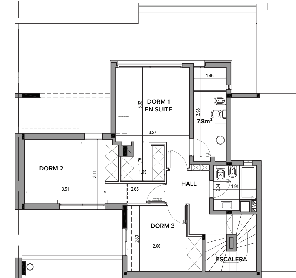
NIVEL 1 69m 2 construidos
