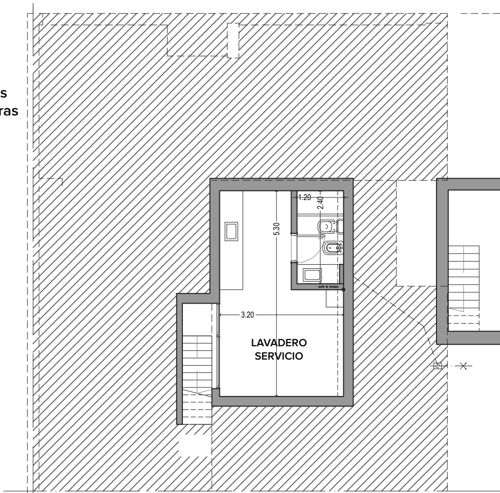
SUBSUELO 21.5m 2 construidos
